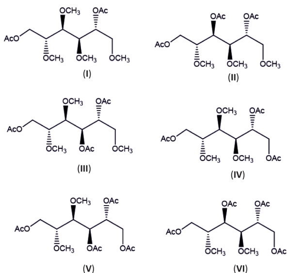
Рис. 5. Перметилированные альдитолацетаты: 1,5-ди- O -ацетил-2,3,4,6-тетра- O -метил-глюцитол (I); 1,3,5-три- O -ацетил-2,4,6-три- O -метил-глюцитол (II); 1,4,5-три- O -ацетил-2,3,6-три- O -метил-глюцитол (III); 1,5,6-три- O -ацетил-2,3,4-три- O -метилглюцитол (IV); 1,4,5,6-тетра- O -ацетил-2,3-ди- O -метилглюцитол (V); 1,3,5,6-тетра- O -ацетил-2,4-ди- O -метил-глюцитол (VI).
